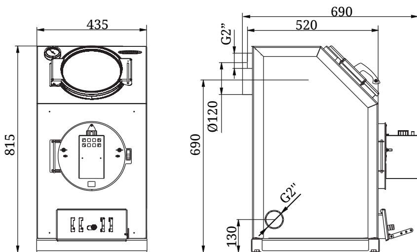
Рисунок 1. Габаритно-монтажные размеры котла «Прагматик 20 Газ»
